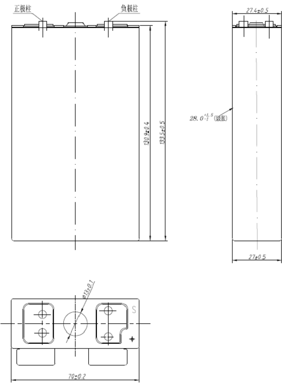
图 1 电池简易外形图
