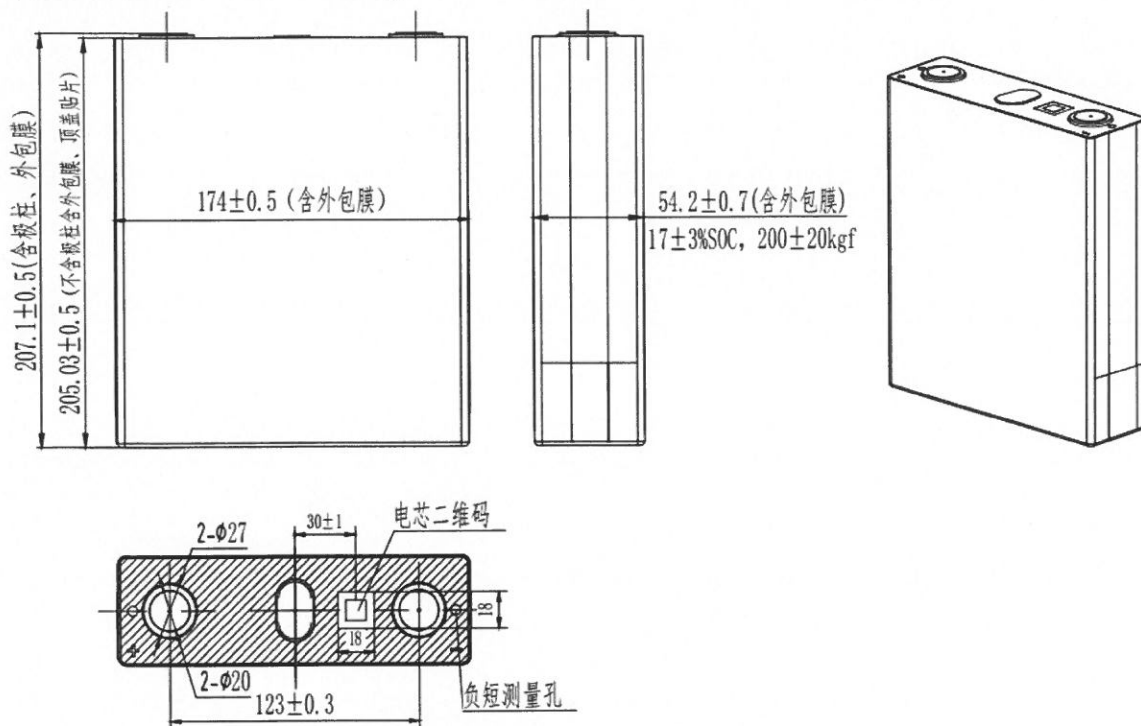
电芯整体尺寸 Cell Dimension
